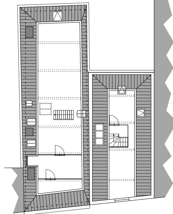
DERDE VERDIEPING bestaande situatie
