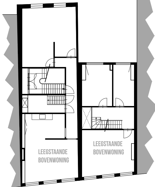
TWEEDE VERDIEPING bestaande situatie
